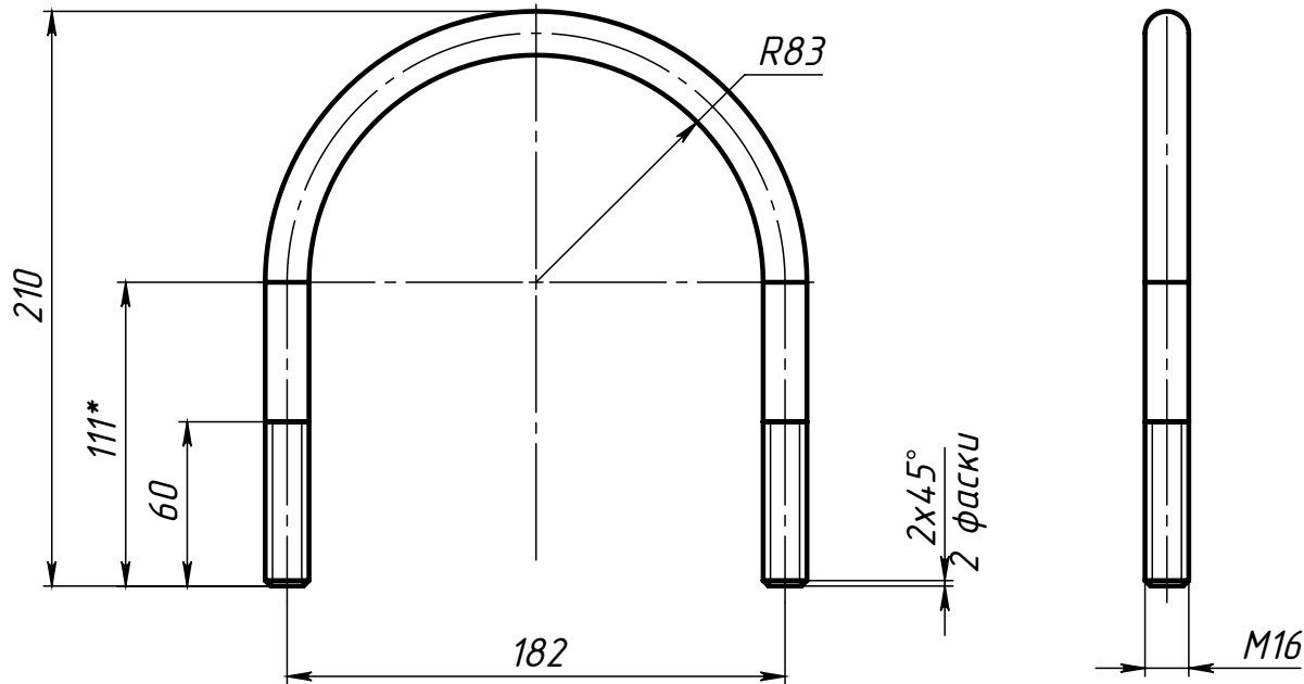
Поз.1 (Хомут)
