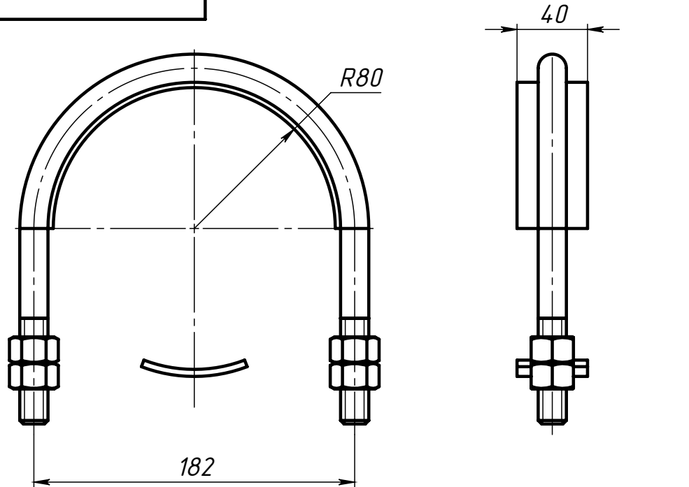
Поз.1 (Хомут)
