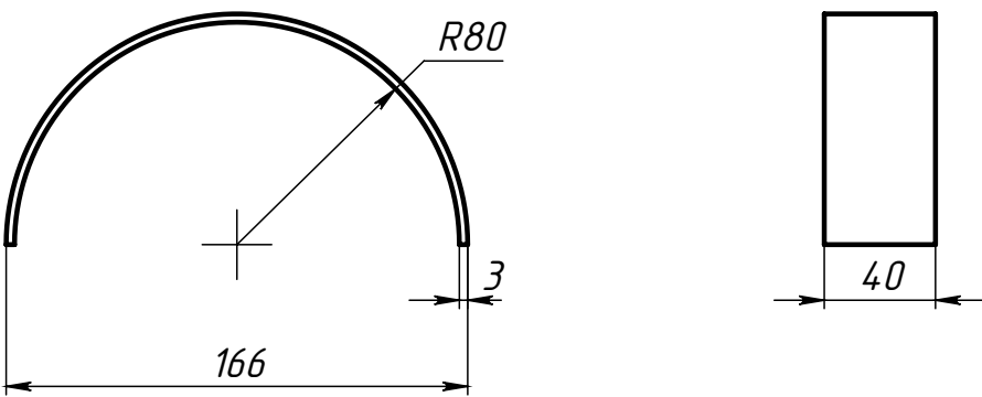
Поз.3 (Прокладка)
